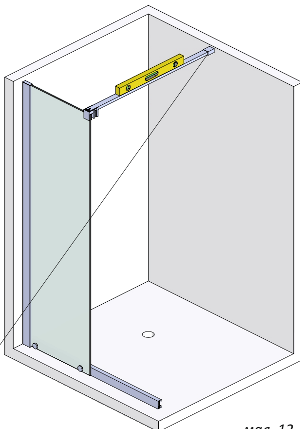
мал. 12 (вигляд спереду)
