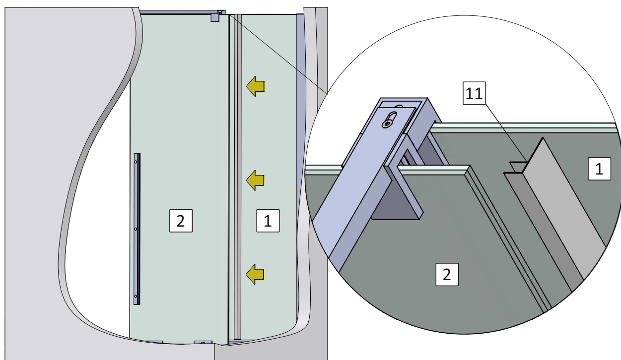
мал. 21 (вигляд ззаду)
