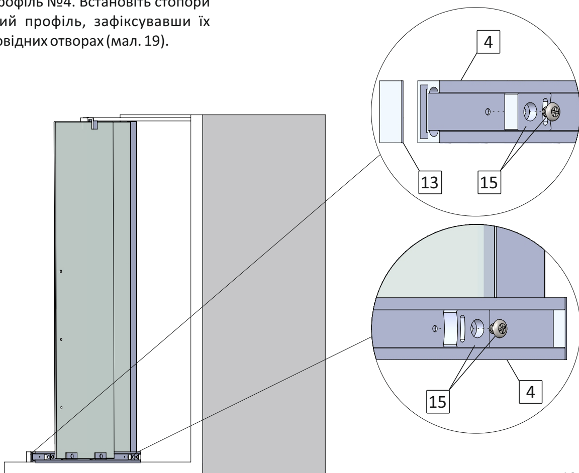
мал. 19 (вигляд ззаду)
