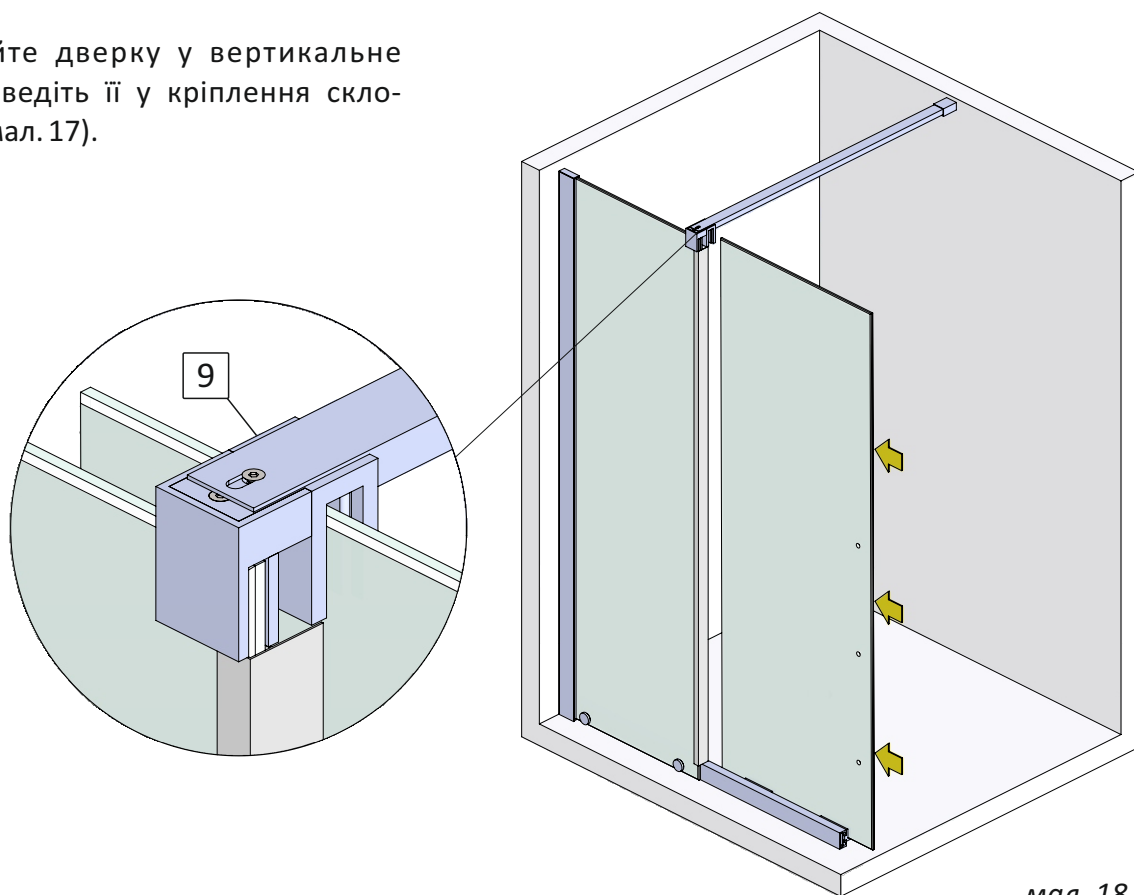
мал. 18 (вигляд спереду)
