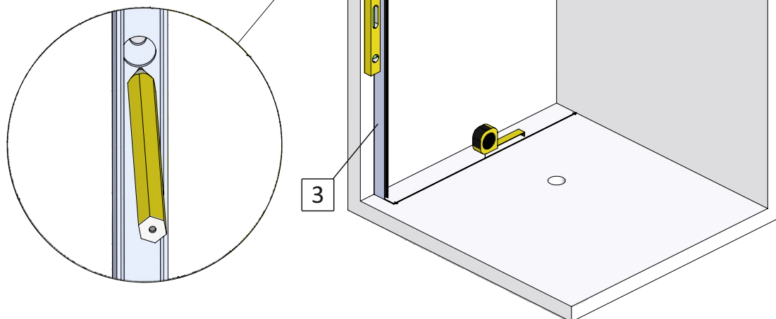
мал. 1 (вигляд спереду)
