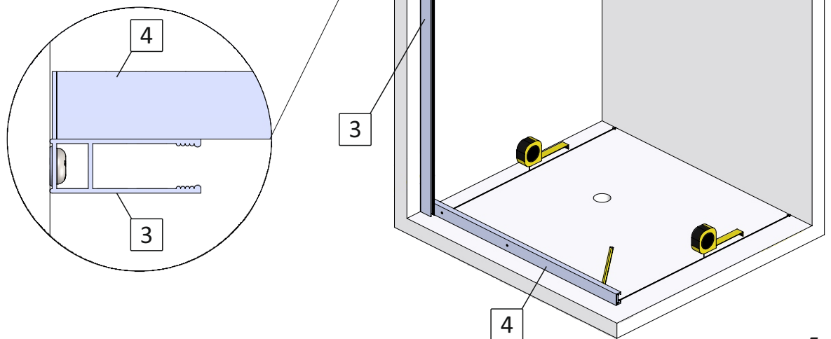
мал. 5 (вигляд спереду)
