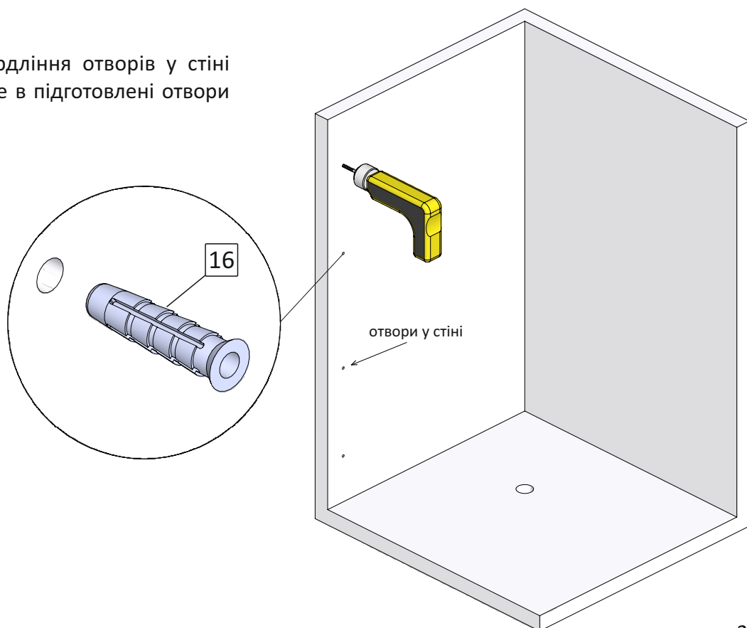
мал. 2 (вигляд спереду)
