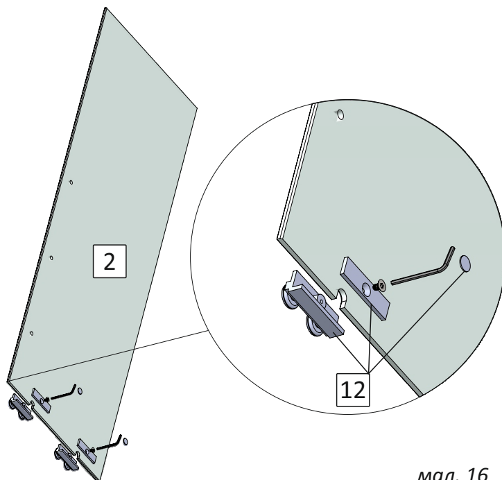
мал. 16 (вигляд ззаду)
