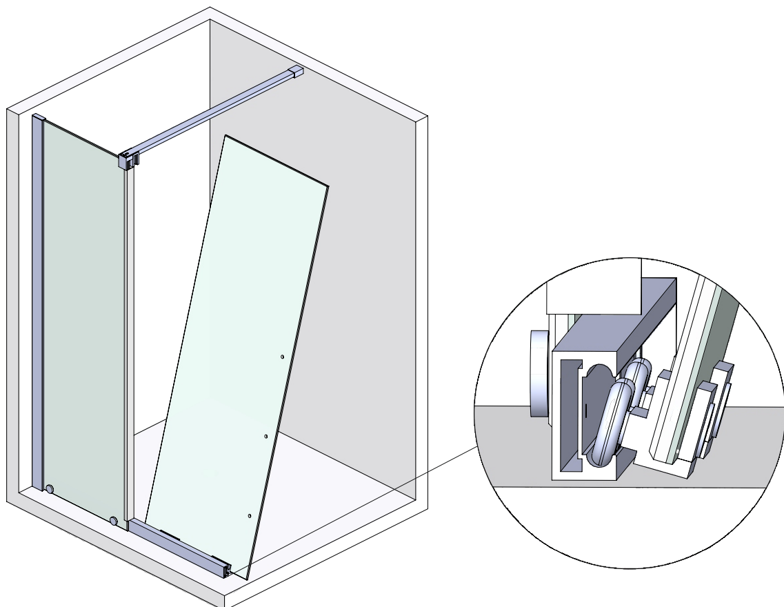
мал. 17 (вигляд спереду)
