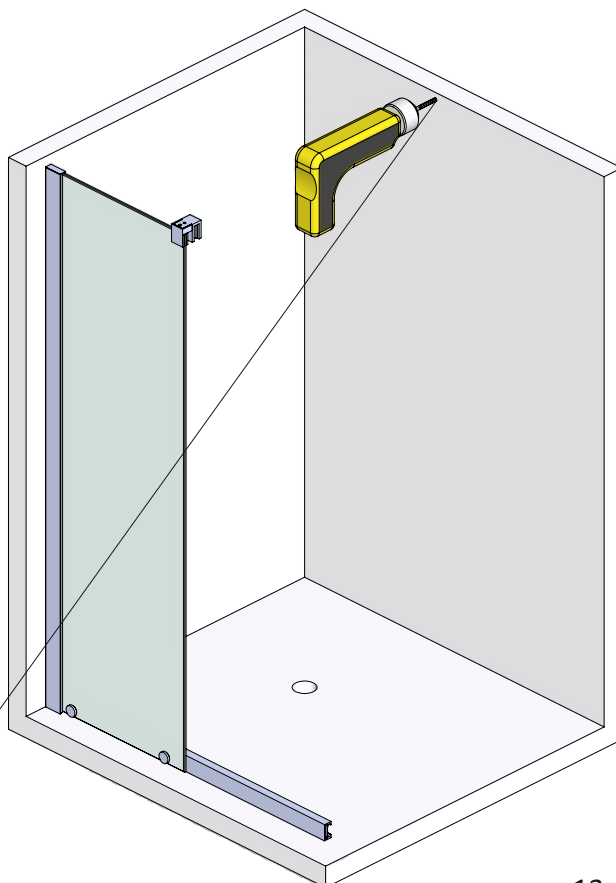
мал. 13 (вигляд спереду)
