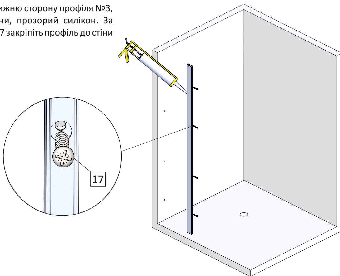
мал. 3 (вигляд спереду)
