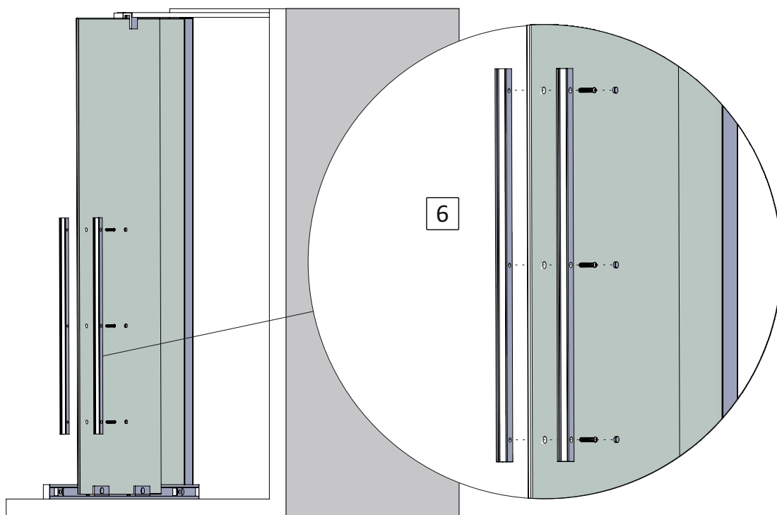
мал. 20 (вигляд ззаду)
